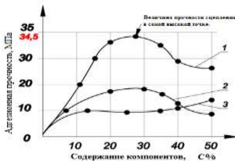
Рис. 3. Зависимость адгезионной прочности композиционного лакокрасочного покрытия от содержания компонентов (а) и времени (в)
