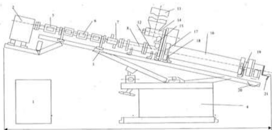
Рис. 1. Устройство для высокочастотной обработки минеральных наполнителей
