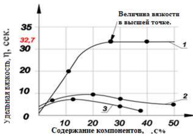
Рис. 4. Зависимость вязкости композиционного лакокрасочного покрытия от содержания компонентов
